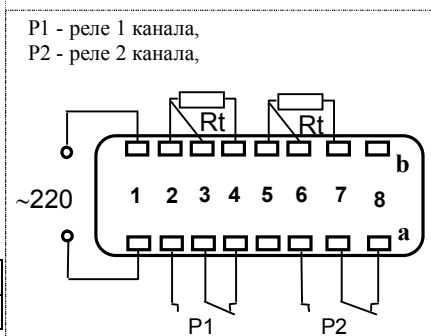
Рис.2-2 Исполнение с разъемом РП14-16
