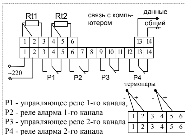
Рис.2-1 Исполнение с клеммными колодками (допускается поставка приборов с реле Р2 и Р4 с двумя выводами 6-7, 12-13)
